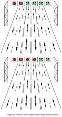
Dispozitive luminoase pentru dirijarea circulației pe benzi reversibile
